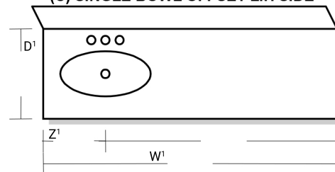
(D) SINGLE BOWL OFFSET R.H SIDE
